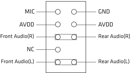
Descrizione prese scheda madre
